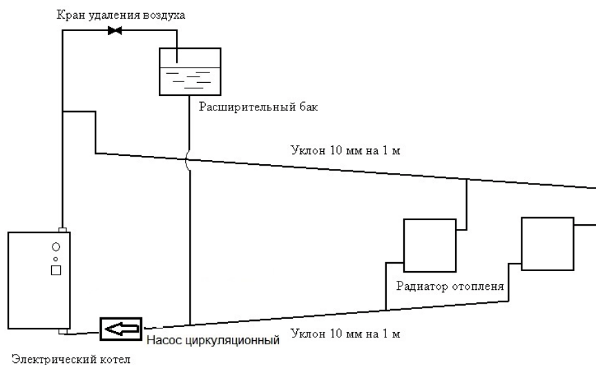
Рис. 4 – Установка электрического котла с открытой системой отопления
