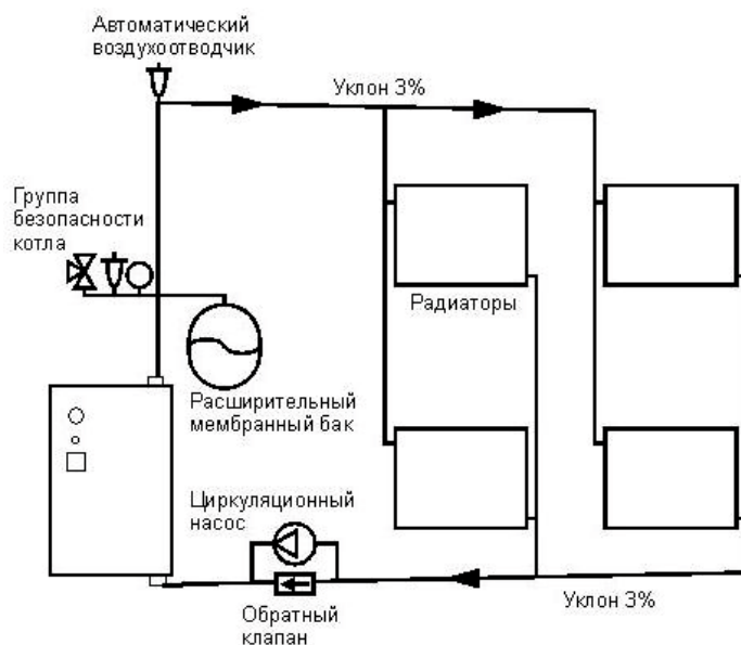
Рис. 5 – Установка электрического котла с закрытой системой отопления
